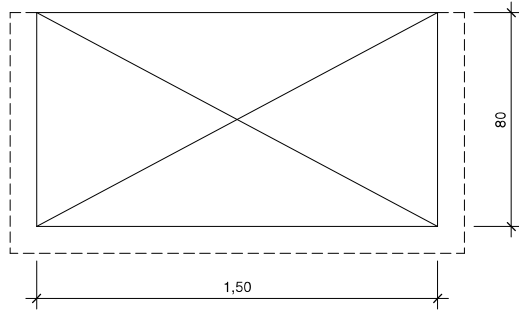
Draufsicht, M1:20
