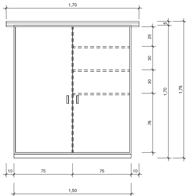
Vorderansicht, M1:20
